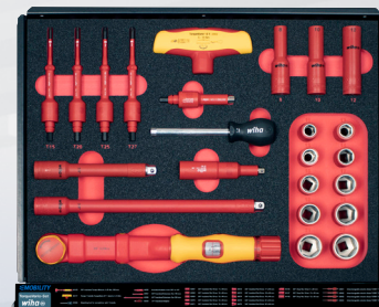
TorqueVario®-készlet
